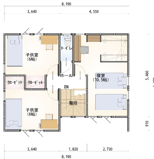
2階 平面図 S:1/80
