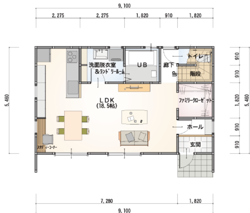
1階 平面図 S:1/80
