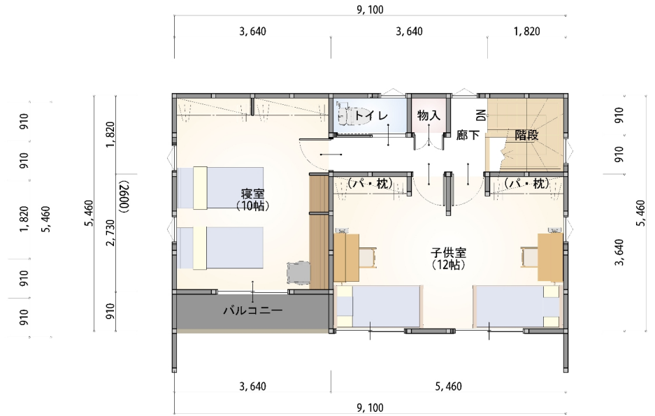
2階 平面図 S:1/80
