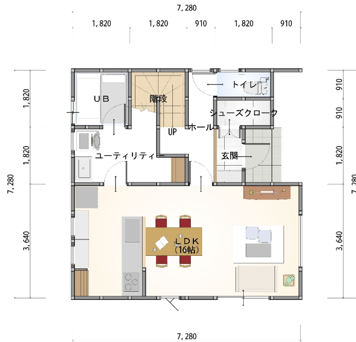
1階 平面図 S:1/80
