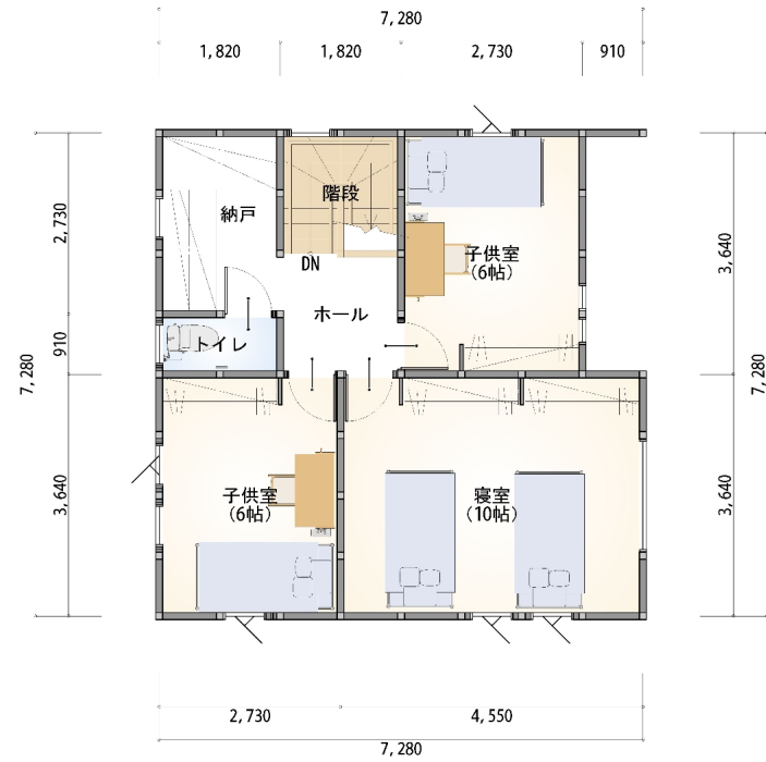
2階 平面図 S:1/80
